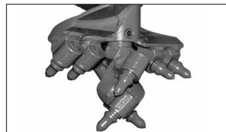
PUNTA ELICOIDALE con doppia elica, taglienti con picchi al Widia per lavoro su asfalto o roccia friabile per mod. TR 100/180/300/600/1200/1500.
